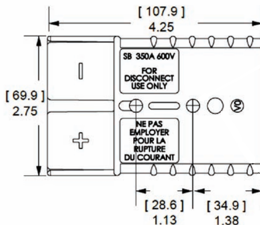
SB350
